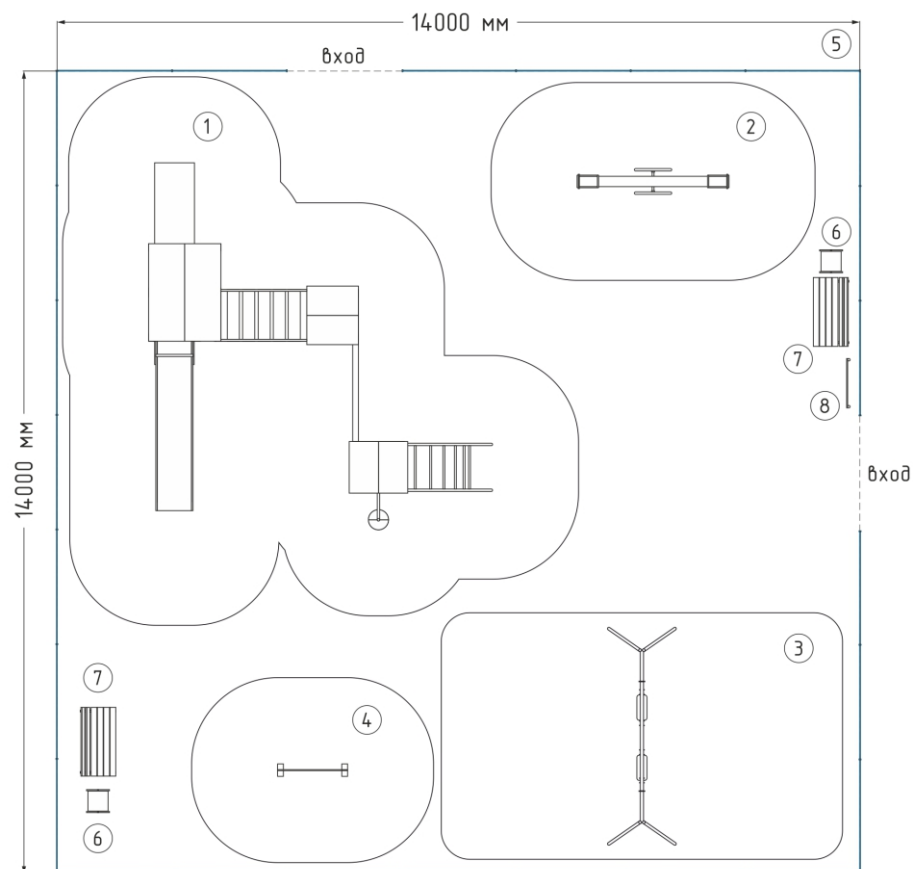
Схема «План сверху» с зонами приземления
